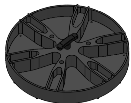
*Plateau - 12 poches Pièces Ømax 20 mm Profondeur 50 mm
